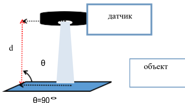
Рисунок 3 - Размещение датчика
