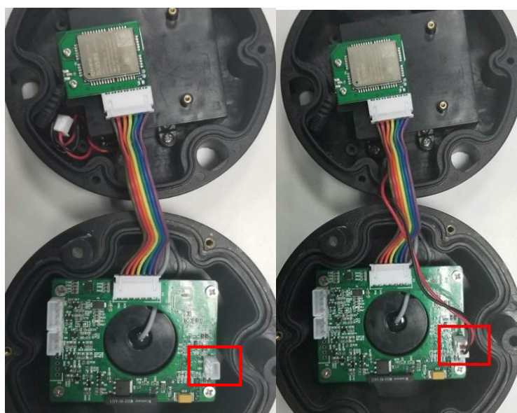
Рисунок 4 - Подключение аккумуляторной батареи
